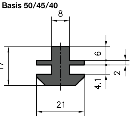
Basis 50/45/40 mit Versatz
