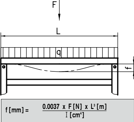
Belastungsfall 4
