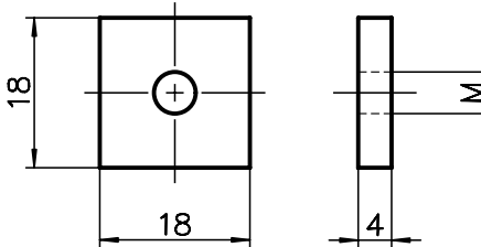
Profil Basis 50 / 45 / 40
