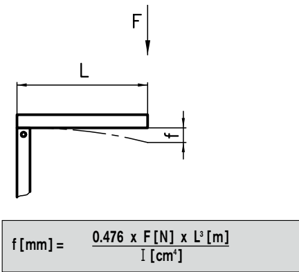
Belastungsfall 1
