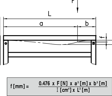
Belastungsfall 3
