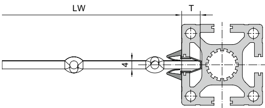
Anwendung mit Einfassprofil C39-70
