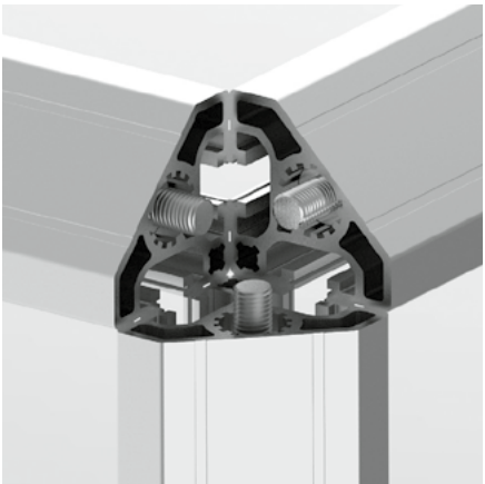
Eckelement-Befestigungssatz 3 Gewindeverbinder
