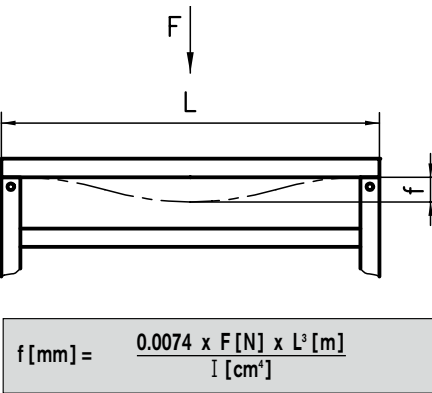
Belastungsfall 2
