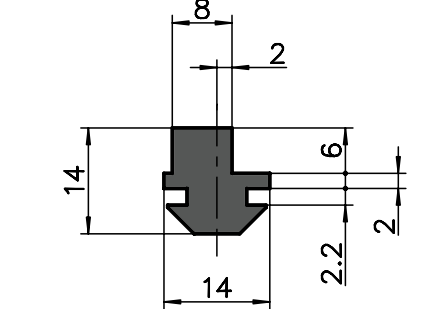
Basis 30/20 mit Versatz
