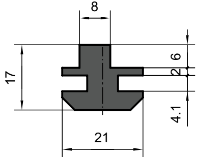
Basis 50/45/40 mit Versatz
