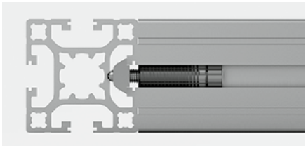
Raccord intégré
