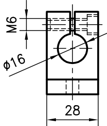
Etrier à 90°
